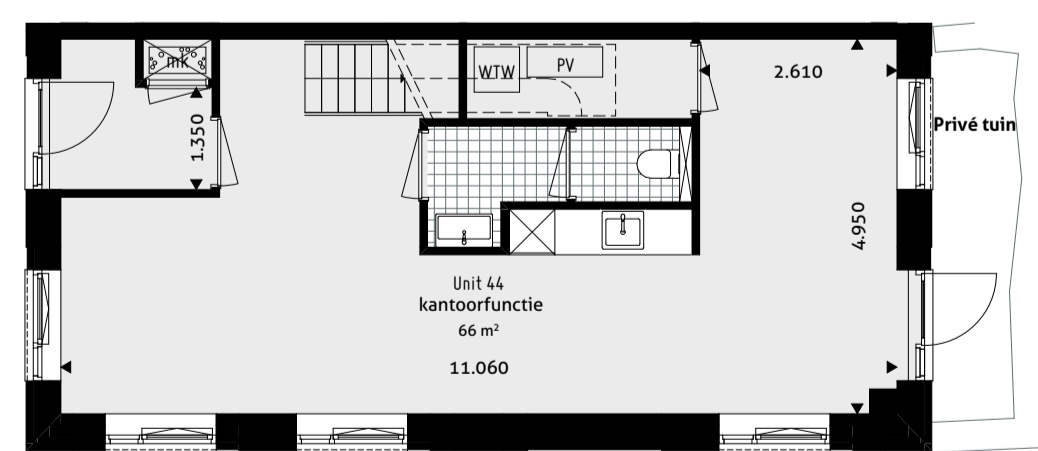
Begane grond 1:100
