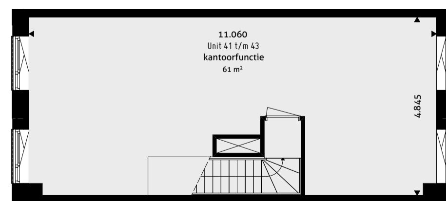
Eerste verdieping 1:100
