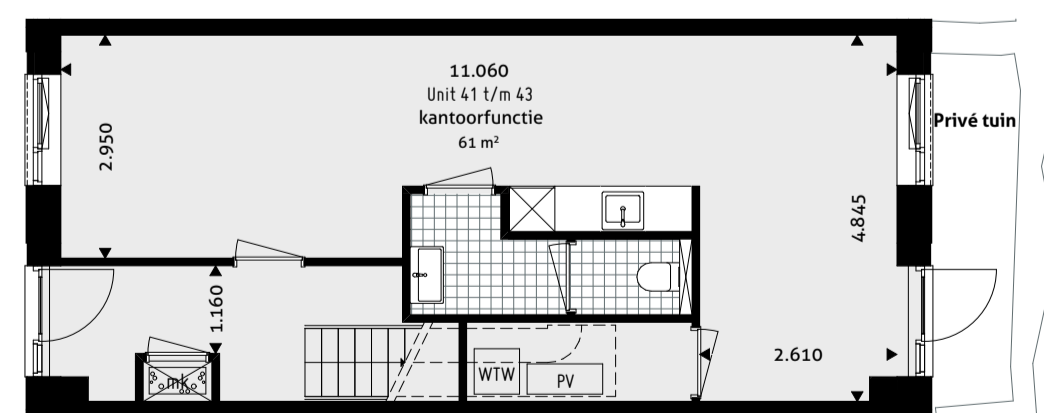
Begane grond 1:100
