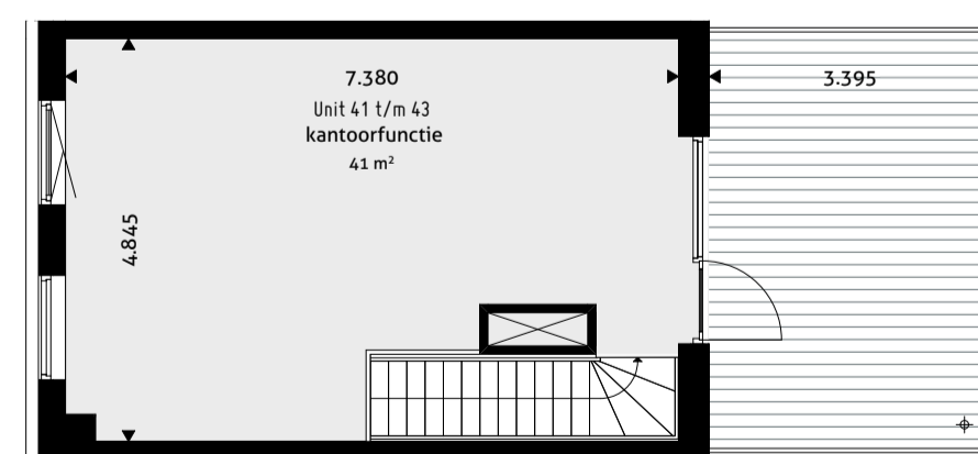
Tweede verdieping 1:100
