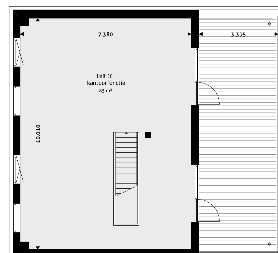
Tweede verdieping 1:100
