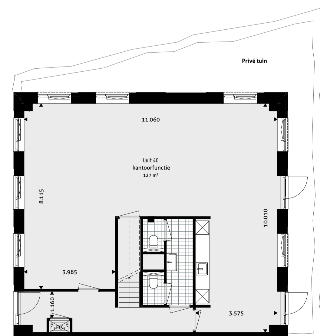
Begane grond 1:100
